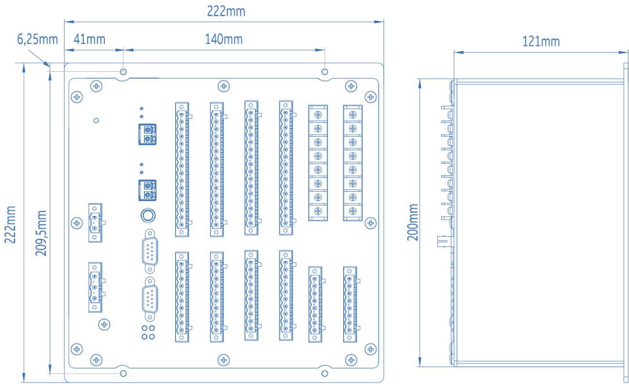
MU320E Dimensions
