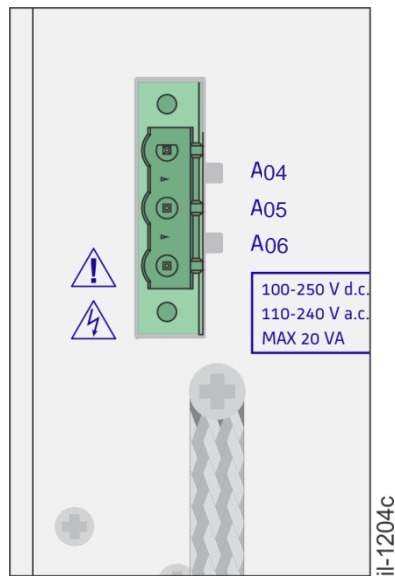
MU320E Earthing
